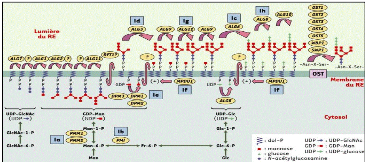
Figure 03. Schéma illustrant le mécanisme de la Nglycosylation des protéines dans le réticulum endoplasmique granuleux.
